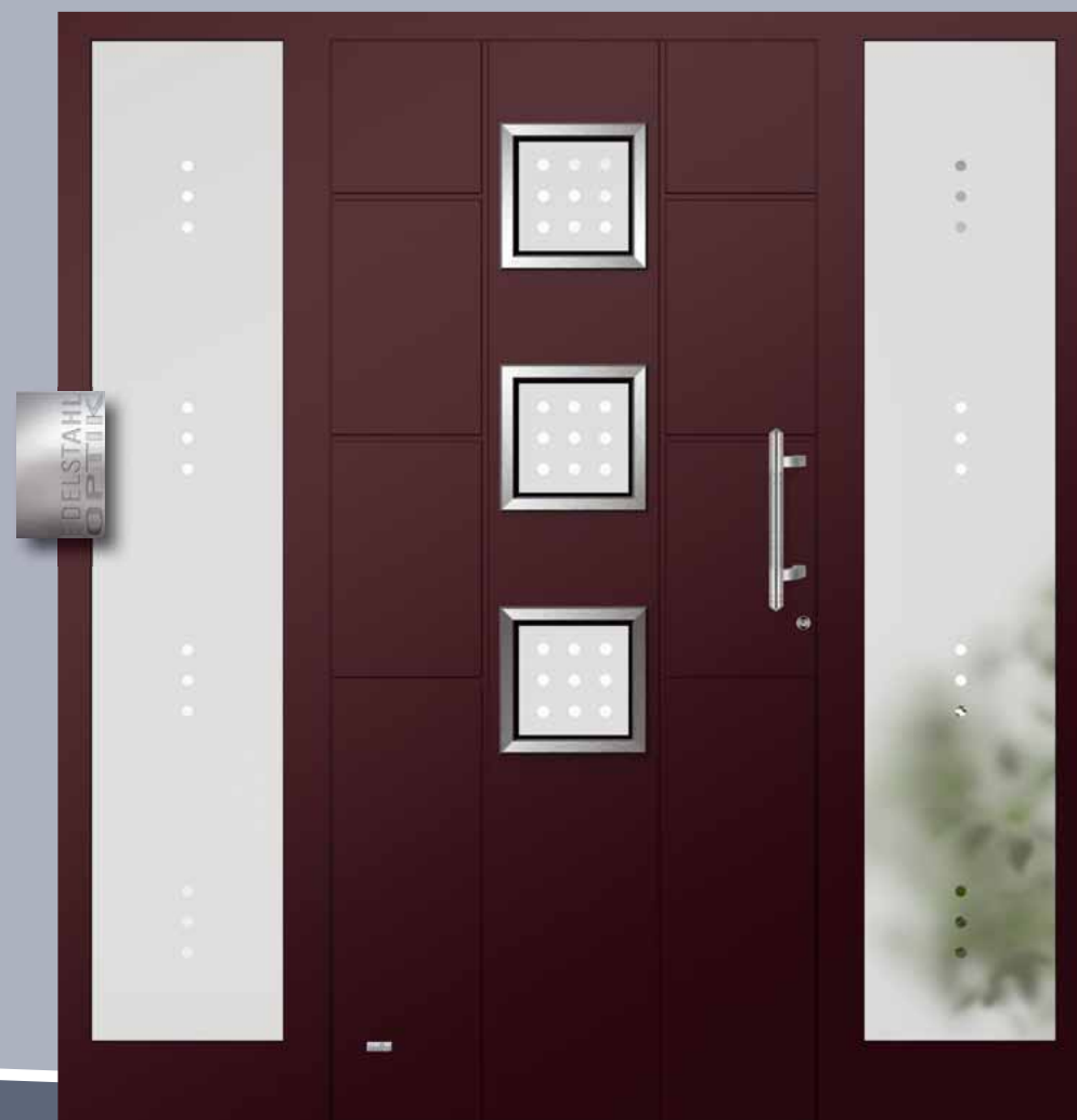
S 1017 geätzt, außen aufgesetzt, RAL 3007 schwarzrot matt / Edelstahl-Optik Glas 1G003 (Float teilmattiert), Griff 1936 Edelstahl
