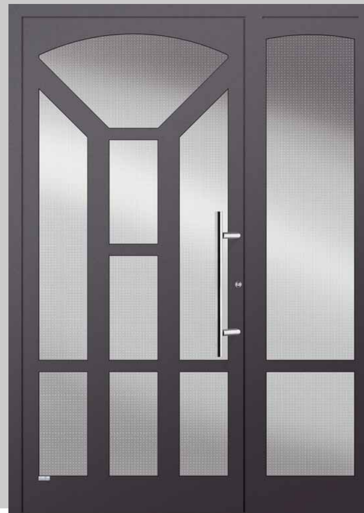
T 520 verschweißt , PLF95 schwarzgrau feinstruktur Glas Mastercarre weiß, Griff 1982 Edelstahl 600 mm
