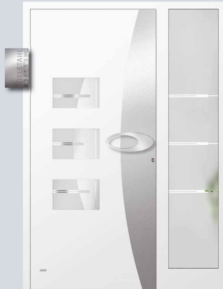
S 3069 außen aufgesetzt, RAL 9016 weiß / Edelstahl-Optik Glas 3U008 (Float in unterschiedlicher Intensität teil mattiert) Griff 1732 Edelstahl
